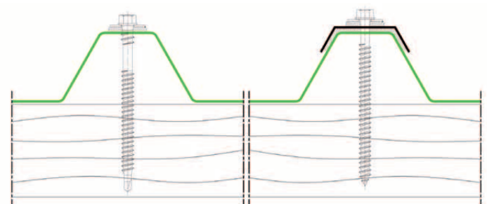
Befestigung ohne Kalotte mit Bohrschraube SXCW (Stützgewinde)
