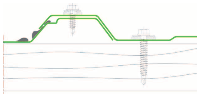
Längsstoß mit Wasserfalle
