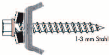
TDA-S-S16-6,5x90 bis 120 mit Kalotte
