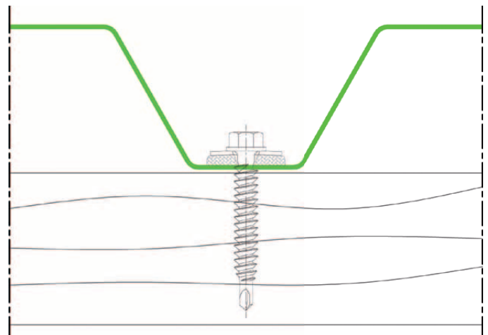
Standard-Verschraubung
