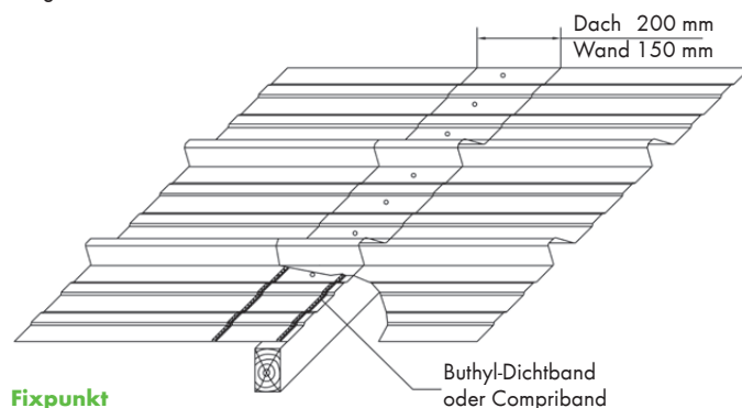
Längsstoß mit Wasserfalle
