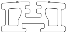
Terrafina UK Riegel . Höhe 35 mm Breite 80 mm
