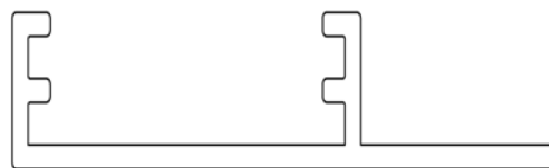
Plattenanker Länge 300 mm Breite 138 mm
